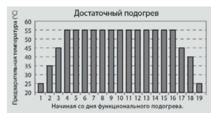
Рис. 16. Достаточный подогрев
