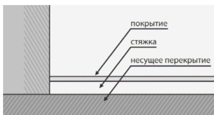
Рис. 13. Соединительная стяжка
