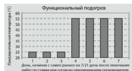
Рис. 15. Функциональный подогрев
